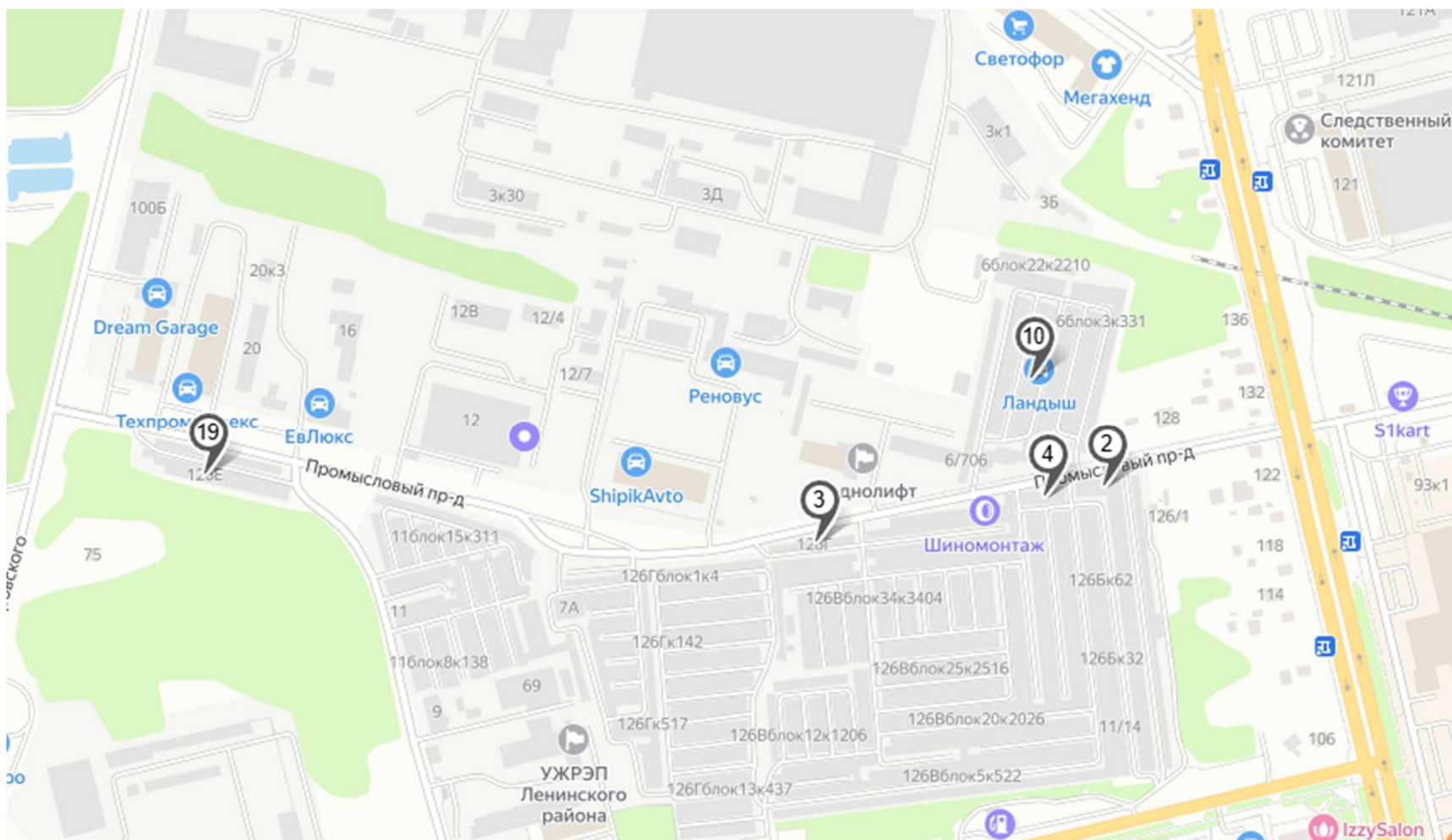
Рисунок 31 – Карта-схема расположения пунктов сбора изношенных шин (2)*
